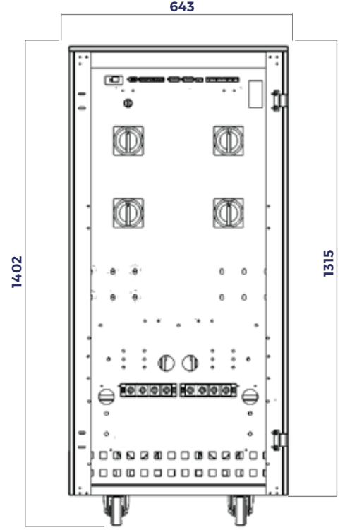
3.3.2 200 kVA U2//U3 Model Ölçüleri (mm)
